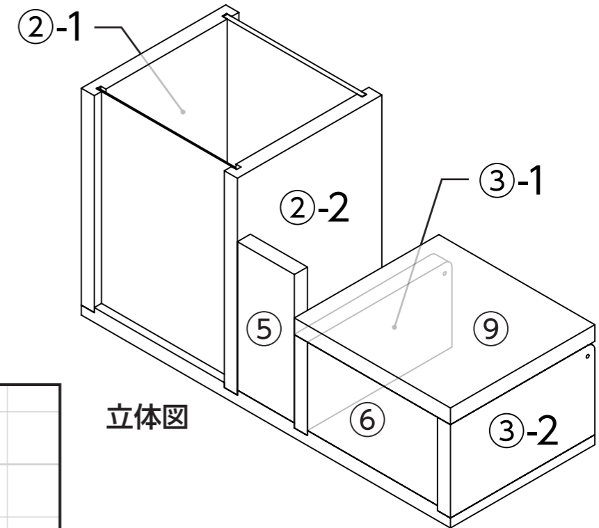
⑤前板A (着色のみ)
